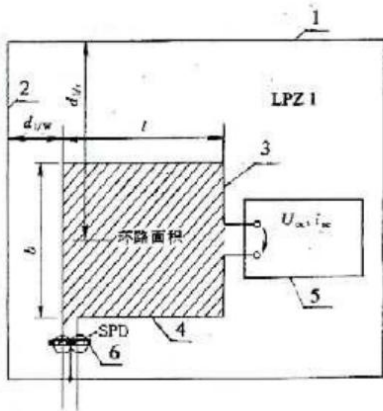
图 G 环路中的感应电压和电流
