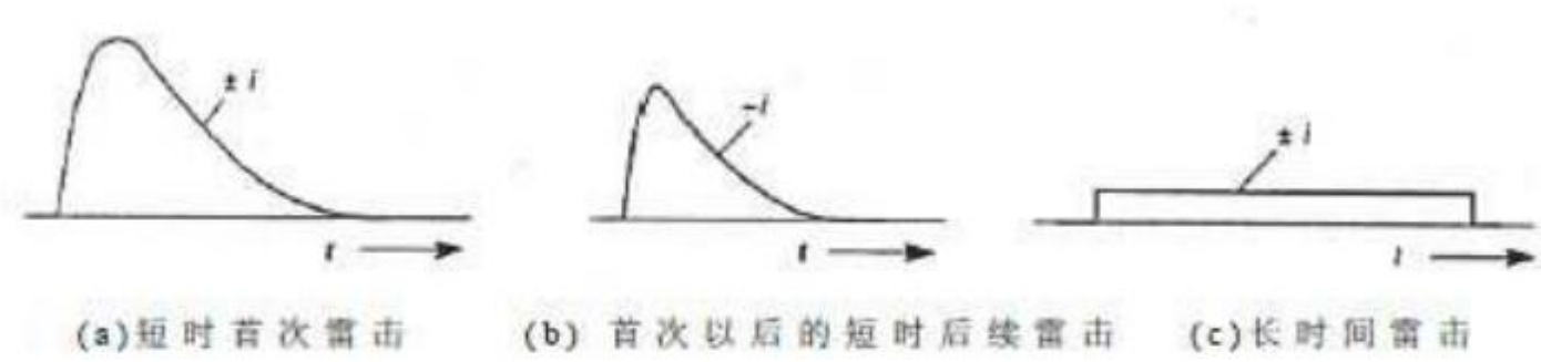
F.0.1-1 闪电中可能出现的三种雷击
